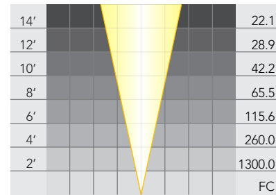
PAR 36 Halogen: LN-7610
