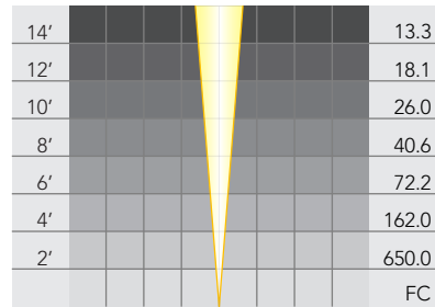
PAR 36: LN-25 NSP
