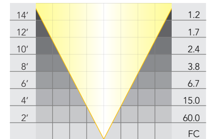
PAR 36: LN-50 VWFL
