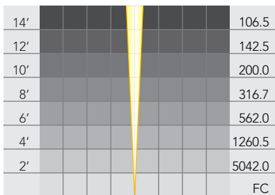
PAR 36 Halogen: LNH-35 VNSP
