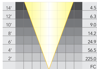
PAR 36 Halogen: LNH-35 WFL
