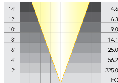
PAR 36: LN-50 WFL
