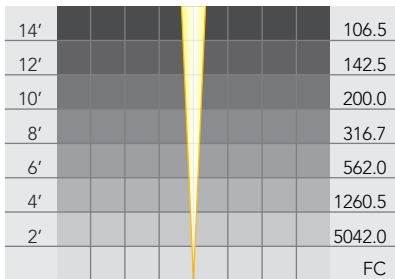
PAR 36: LN-50 VNSP
