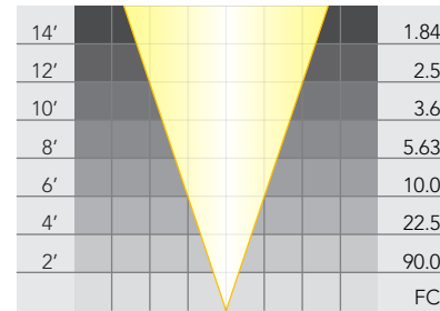
PAR 36: LN-25 WFL
