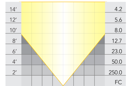
PAR 36 Halogen: LN-7606
