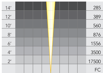
PAR 36 Halogen: LN-7616
