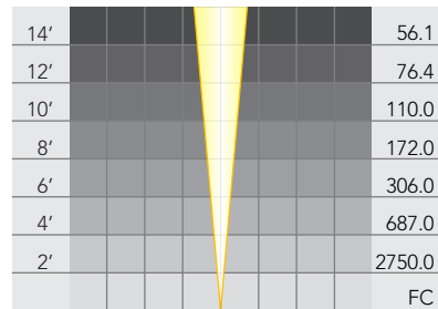
PAR 36: LN-50 NSP
