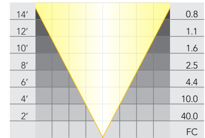
PAR 36: LN-25 VWFL
